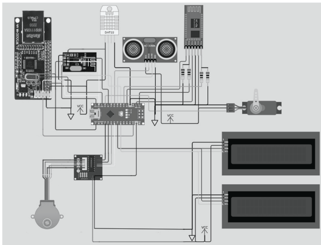
Рис. 3. Схема підключення сенсорів і актуаторів до Arduino NANO №2
